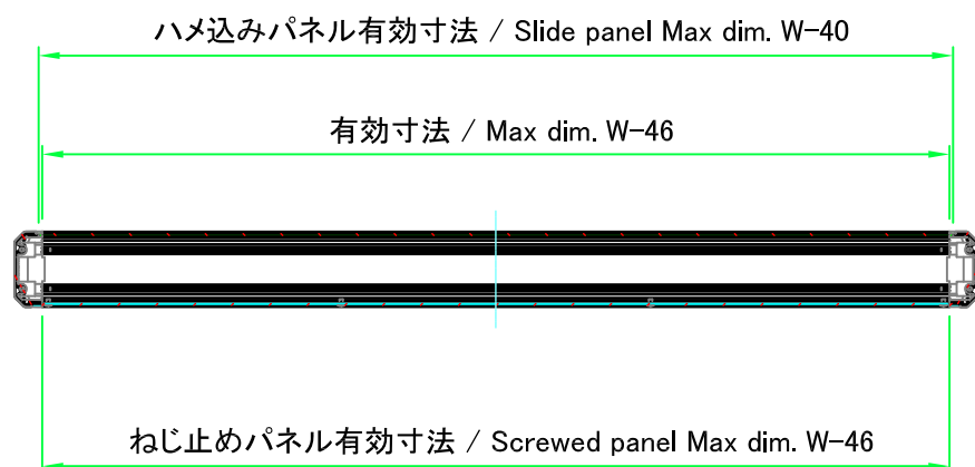
A-A ( 1 : 7 )
